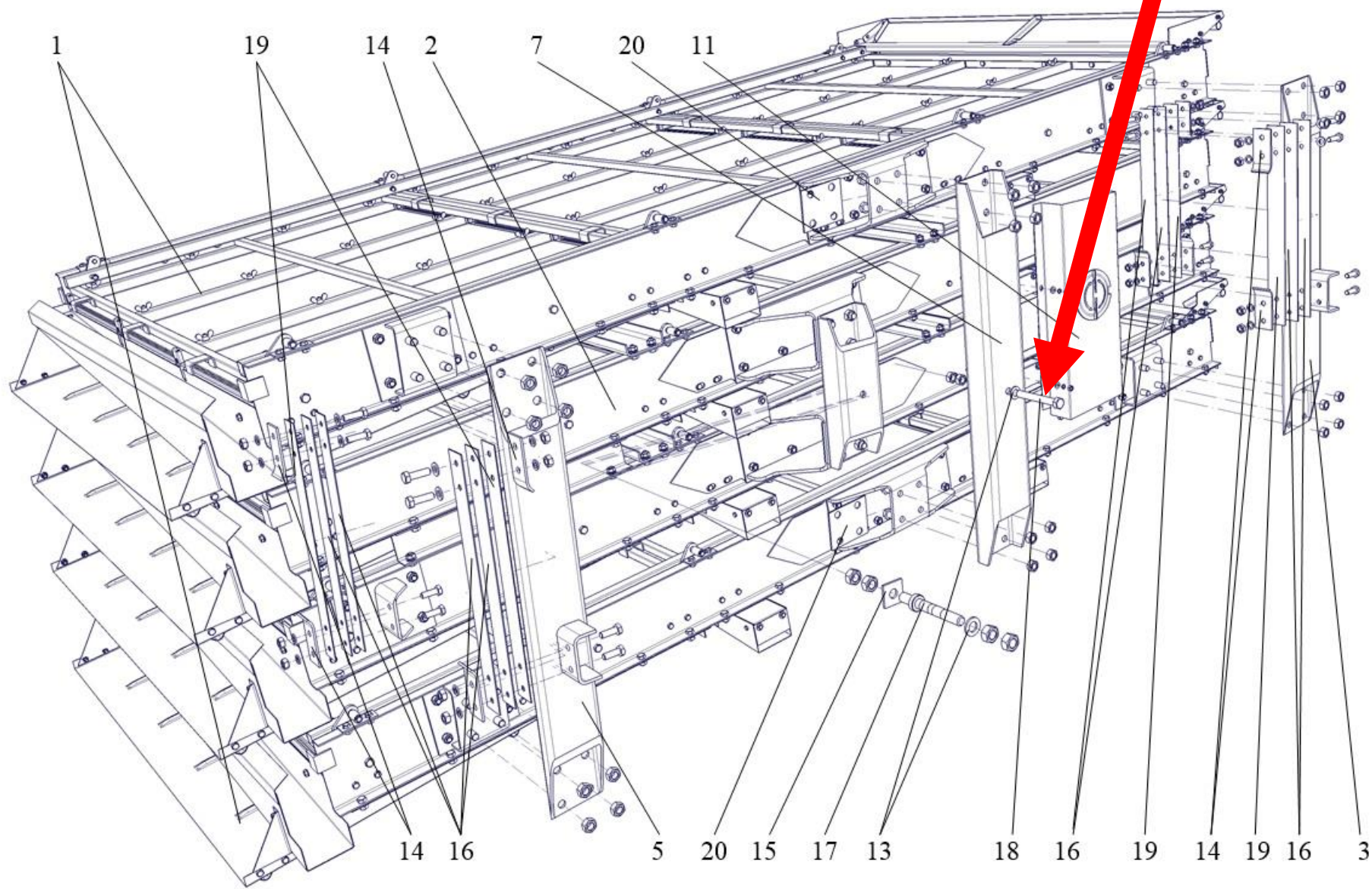
Рис. 12 СВУ60.07.000А
